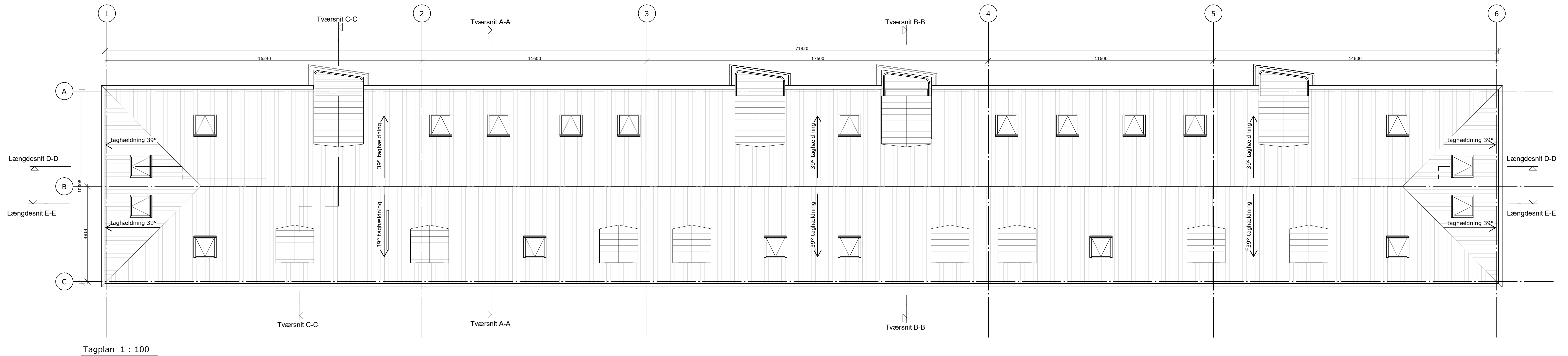
Tagplan 1 : 100
